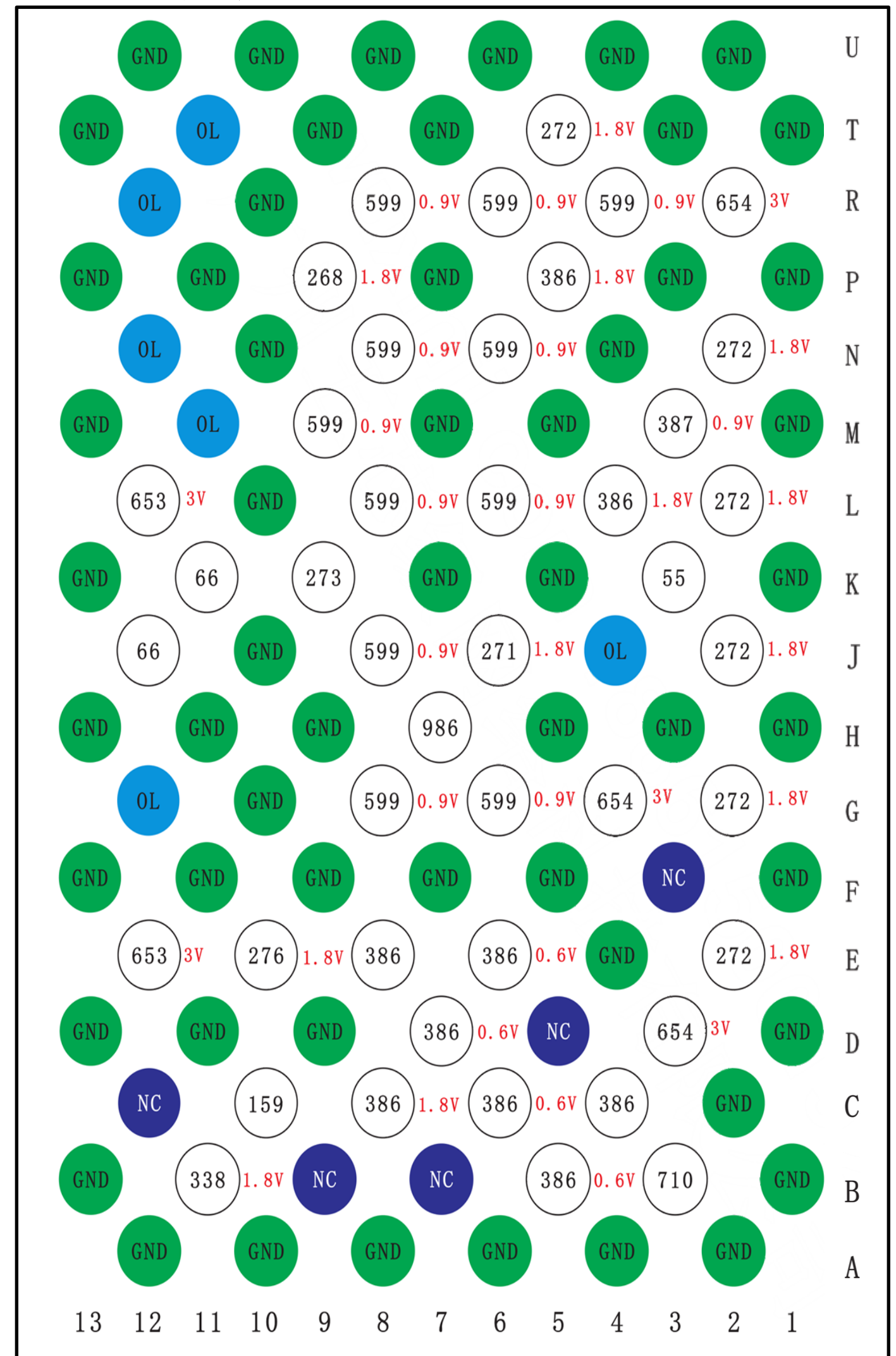
iPhoneX U2600硬盘对地阻值图
